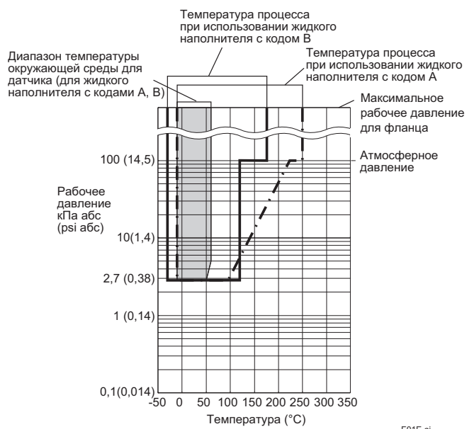
Рис. 1-1. Рабочее давление и температура процесса (Жидкий наполнитель: силиконовое масло для общего применения)
